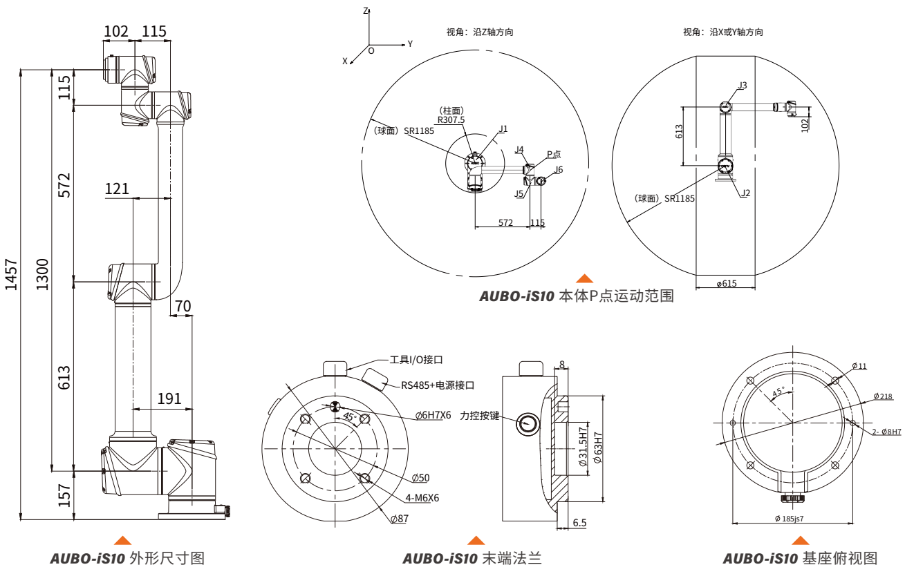
iS10 尺寸图
