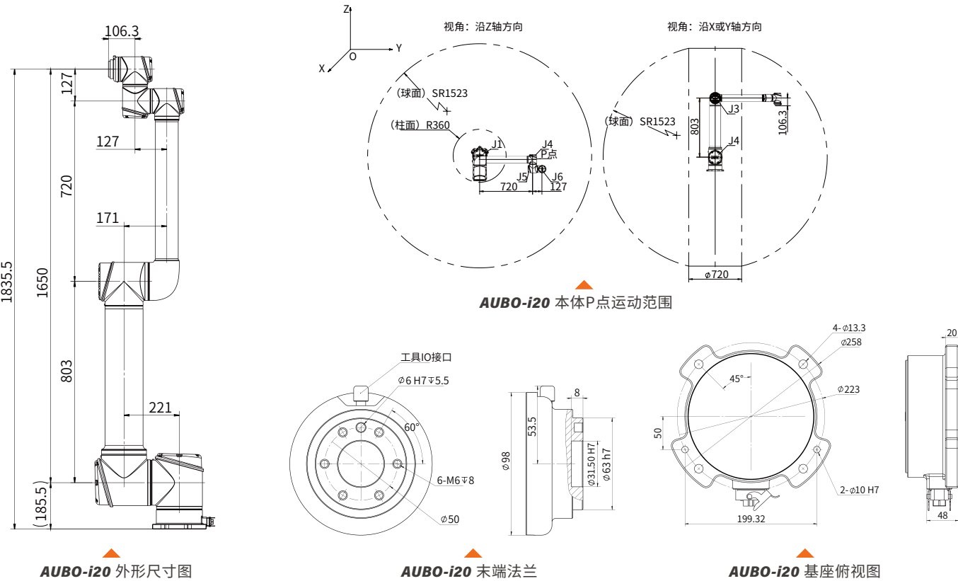
i20 尺寸图
